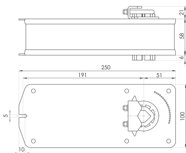
РАЗМЕРЫ мм
